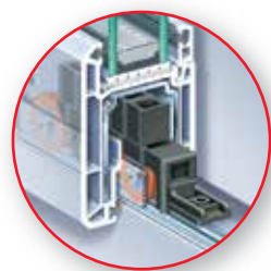
Laufrollen aus speziellem Hart-PVC sorgen für ausgesprochene Laufruhe und Leichtgängigkeit
