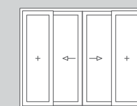
Vierteiliges Element mit zwei Schiebeflügeln und zwei Festverglasungen
